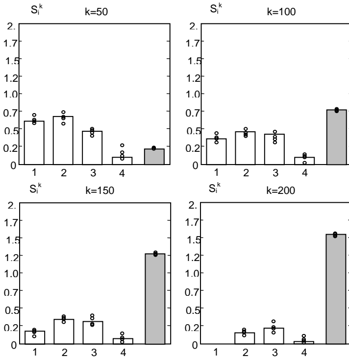
Рис. 3. Опытные и расчетные данные эволюции распределения содержания мелкой фракции по высоте слоя и степень их извлечения в подситовое пространство
