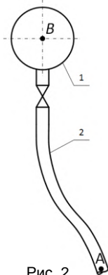
Рис. 2 1 – паропровод, 2 – дренаж
