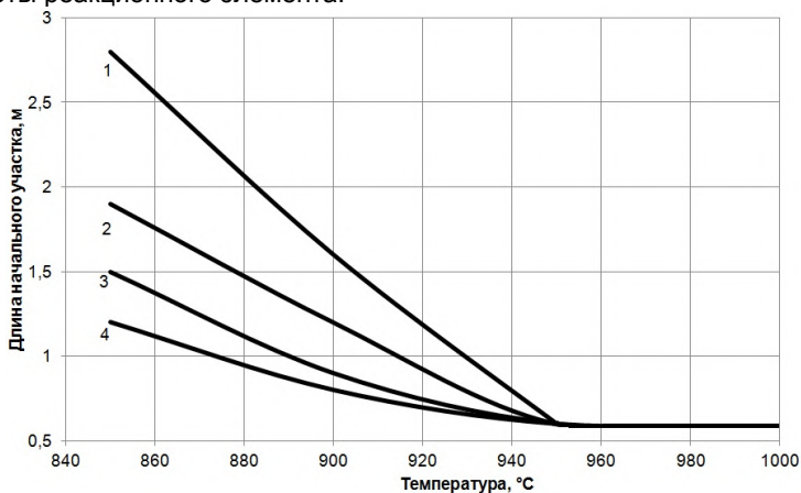
Рис. 2. Зависимость L_{нач} от температуры парогазовой смеси и удельного расхода пара: 1 – V_{пар} = 1,7 ; 2 – V_{пар} = 2,0 ; 3 – V_{пар} = 2,5 ; 4 – V_{пар} = 3,0
