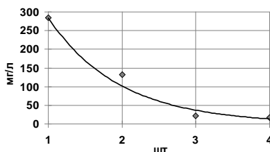
Рис. 2. Зависимость количества вымываемых органических соединений от кратности обработки анионита
