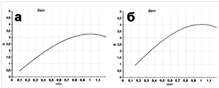
Рис. 2. Графики изменения Gain в зависимости от относительного расхода q/q_m ( q – относительный расход, q_m – максимальный расход в пределах рабочего диапазона РО). Пропускная способность трубопроводной сети – 67,3 \text{ м}^3/\text{час} , диаметр трубы – 170 \text{ мм} .
