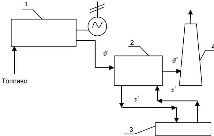
Рис. 1. Принципиальная схема ТЭЦ в составе: ГПГУ и КУ: 1 – газопрошневая генераторная установка (ГПГУ), 2 – котел-утилизатор (КУ), 3 – индивидуальный тепловой пункт (ИТП), 4 – дымовая труба (ДТ); \varphi' = 455^{\circ}\text{C} , \varphi'' = 120^{\circ}\text{C} , t' = 70^{\circ}\text{C} , t'' = 95^{\circ}\text{C} .
