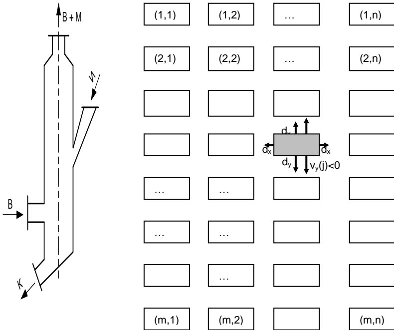
Рис. 1. Конструктивная схема гравитационного классификатора ( B – воздух, I – исходный материал, K – крупный продукт, M – мелкий продукт), двумерная ячеечная модель рабочего объема и возможные вероятности переходов
