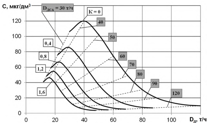
Рис. 2. Основная режимная характеристика вакуумно-атмосферной деаэрационной установки на базе деаэраторов «ДСА» и «АВАКС»: D_d – расход деаэрированной воды потребителям; K – кратность циркуляции; D_{дса} – расход деаэрированной воды ДСА-100
