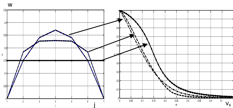
Рис. 2. Влияние профиля скорости (а) на ливные разделения (б)
