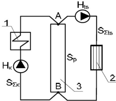
Рис. 1. Принципиальная схема источника теплоснабжения с термогидравлическим распределителем: 1 – источник тепловой энергии; 2 – потребитель; 3 – ТГР
